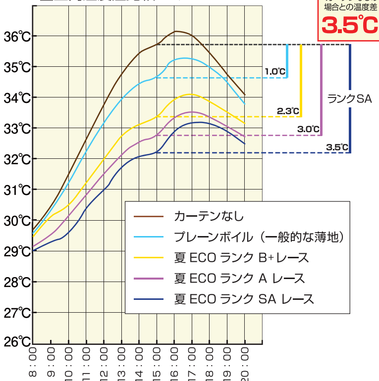
■室内温度差比較シミュレーション
